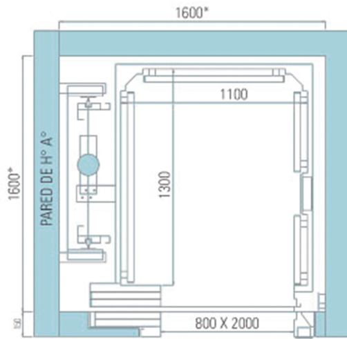
● Pistón Lateral 2:1
