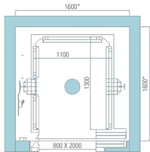
● Pistón Central
