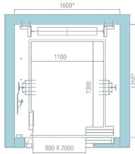
● Cabina tipo 1 - Contrapeso Atrás
