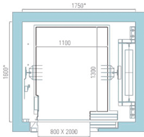
● Cabina tipo 1 - Contrapeso Lateral
