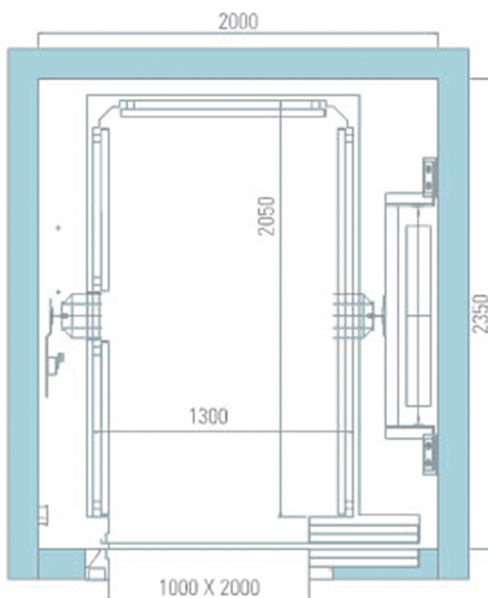
● Cabina tipo 3 - Puerta de 1000mm
