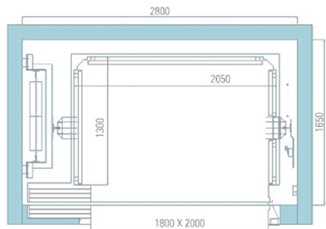
● Cabina tipo 3 - Puerta de 1800mm
